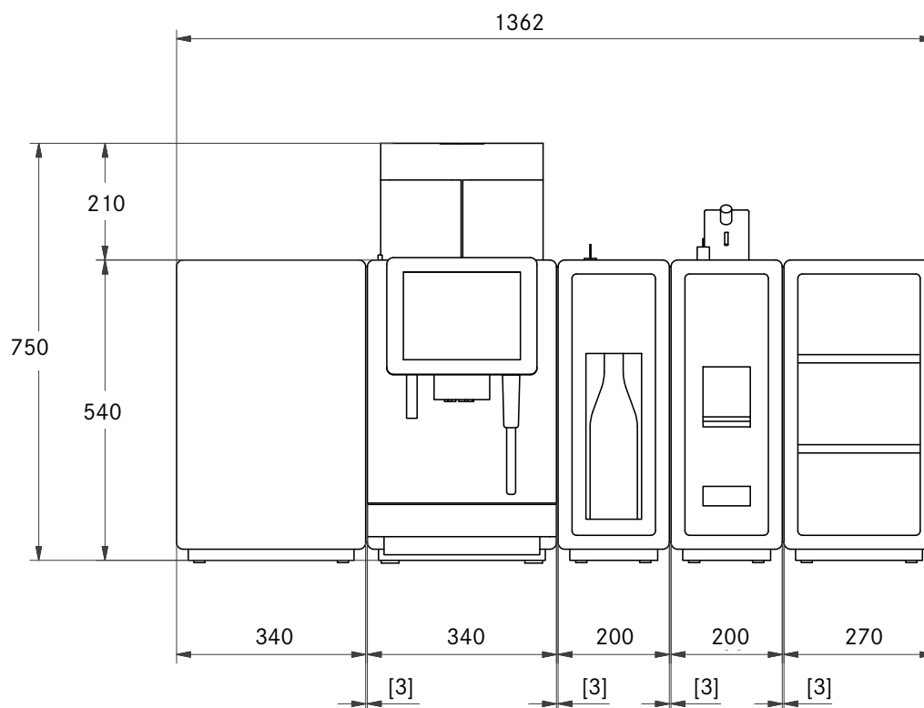
A1000 с SU12 и другим дополнительным оборудованием
