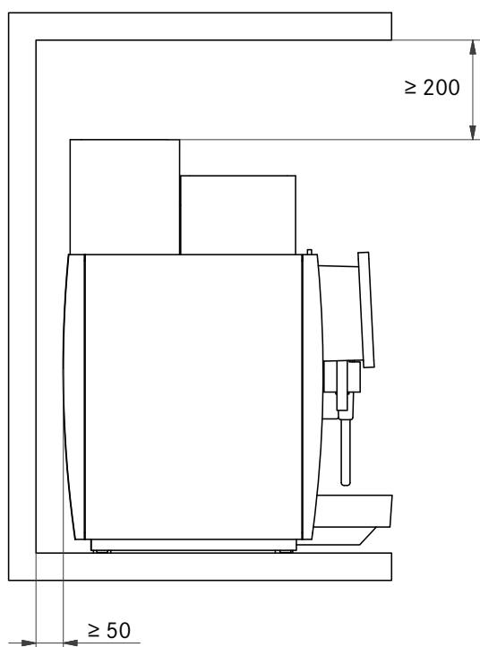
Габаритные размеры на месте установки
